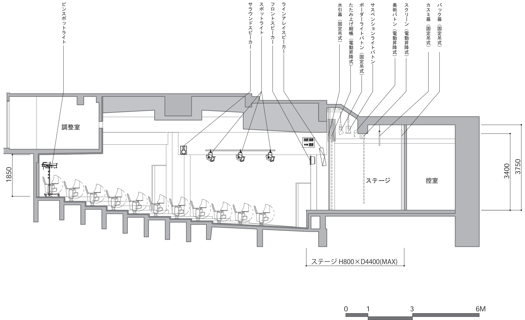
日比谷コンベンションホール(大ホール) 断面図 1/100
